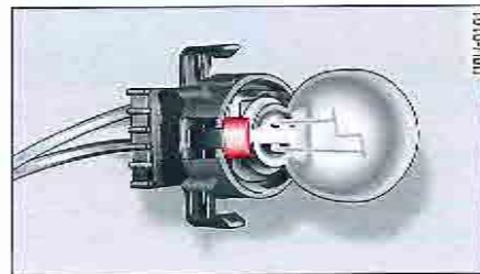
Fig. 214 Douille d'ampoule de clignotant
