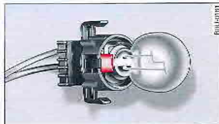
Fig. 212 Douille d'ampoule de clignotant
