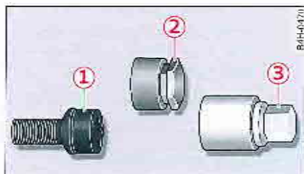
Fig. 193 Boulon de roue antivol avec capuchon de protection et adaptateur
