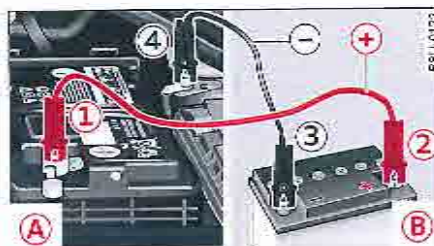
Fig. 194 Compartiment-moteur : raccords de chargeur et de câble d'aide au démarrage
