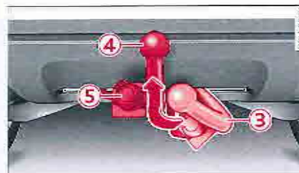
Fig. 158 Pare-chocs arrière : encliquetage du dispositif d'attelage et ouverture de la prise de courant
