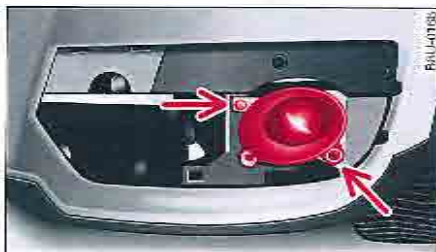
Fig. 217 Phare antibrouillard : vis de fixation.
