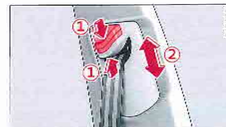
Fig. 143 Dispositif de réglage des ceintures en hauteur pour les places avant - levier de renvoi
