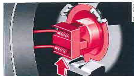
Fig. 206 Connecteur en plastique : dépose du feu de route.
