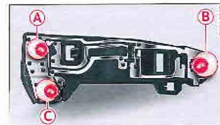
Fig. 221 Feu arrière : support d'ampoules.
