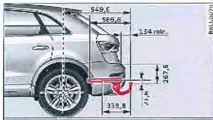
Fig. 160 Emplacement des points de fixation, vue latérale
