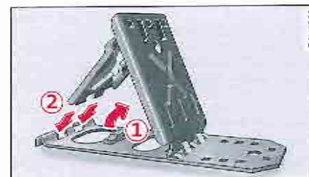
Fig. 180 Déplier les cales repliables
