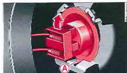
Fig. 207 Connecteur en plastique : repose du feu de route.
