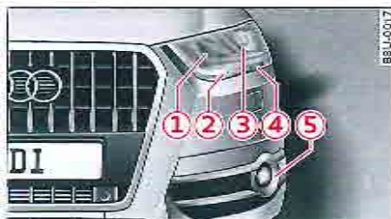
Fig. 201 Phares halogènes : vue d'ensemble côté gauche du véhicule.
