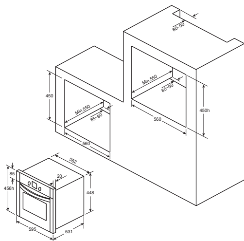
Fig. 5: Distanze di installazione per forni elettrici semplici di 60 cm di ampiezza (la forma della parte superiore può variare) e l'incasso nell'armadio.
