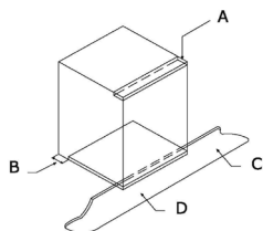
Fig. 7: Requisiti di ventilazione e rifilatura per l'installazione di un forno elettrico semplice in un'unità di cucina standard. Requisiti di ventilazione minimi per gli scaffali superiori, di base e di supporto della parte posteriore dell'unità.
