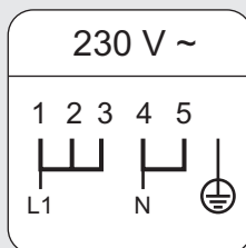
Schéma de branchement
