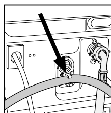
Haak voor een afvoerbuis die op een hoogte van minder dan 60 cm eindigt
