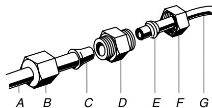
A. Tubería de agua del refrigerador B. Tuerca (provista) C. Bulbo
