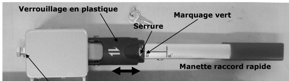
Écrou réglage assemblage express
