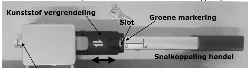
Instelschroef snelkoppeling (inclusief borgmoer)
