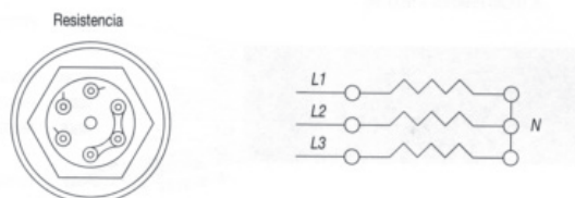
Variante alimentación eléctrica
