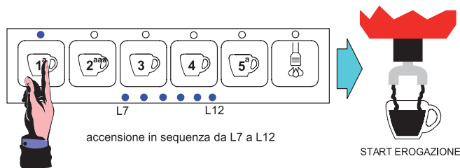
PULSANTIERA 6 TASTI / 12 LED
