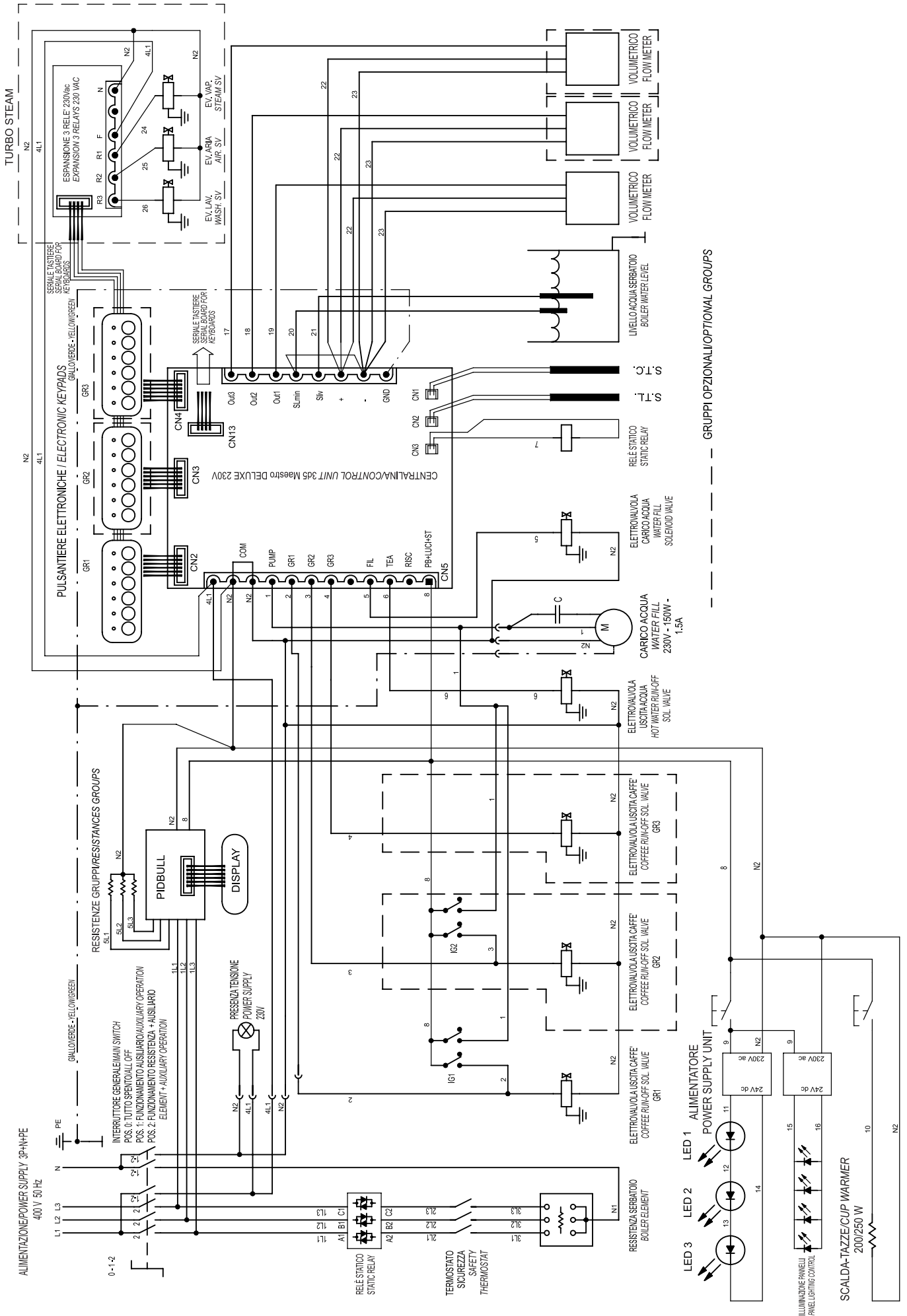
Schema elettrico/Wiring diagram ROMA TCS SED Agg./Update 7/08
