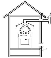
Scarico tramite camino o canna fumaria ramificata (riservata agli apparecchi di cottura)
