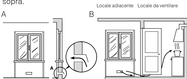
A Apertura di ventilazione per l'aria comburente
