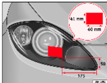
Fig. 156 Phare droit
