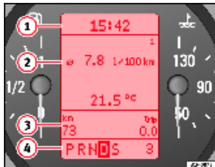
Fig. 38 Afficheur numérique du combiné d'instruments
