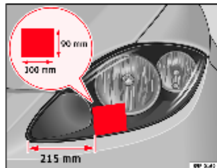
Fig. 151 Phare gauche
