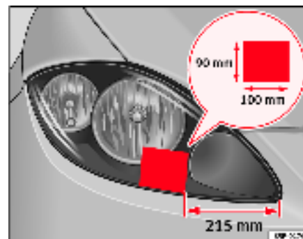
Fig. 152 Phare droit
