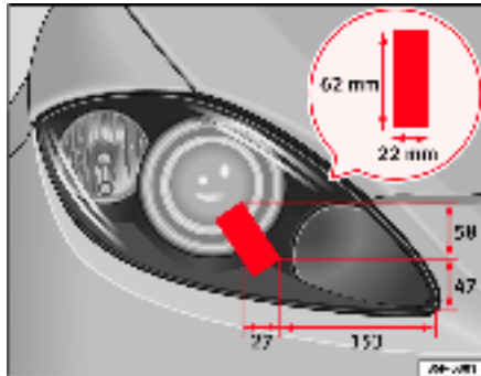
Fig. 154 Phare droit
