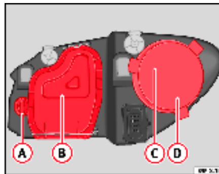
Fig. 182 Lampes du projecteur principal
