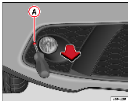
Fig. 205 Accès logement oeillet de remorque
