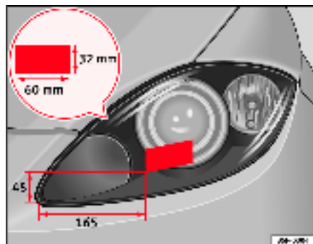
Fig. 157 Phare gauche
