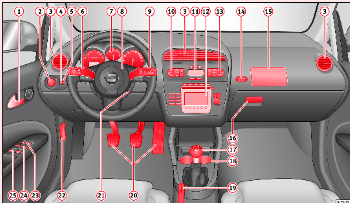
Fig. 32 Tableau de bord
