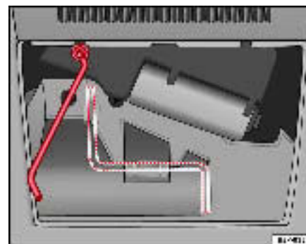
Fig. 72 Manivelle de fermeture d'urgence
