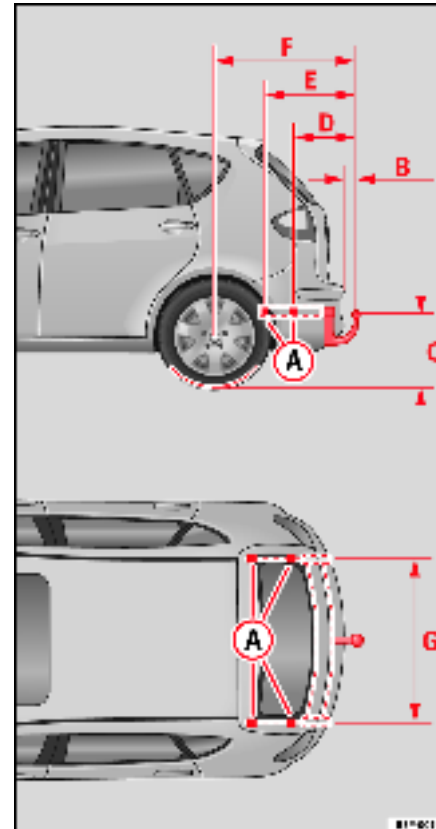
Fig. 158 Points de fixation du dispositif d'attelage
