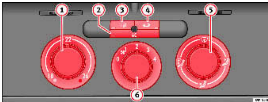
Fig. 129 Sur le tableau de bord : éléments de commande du Climatic
