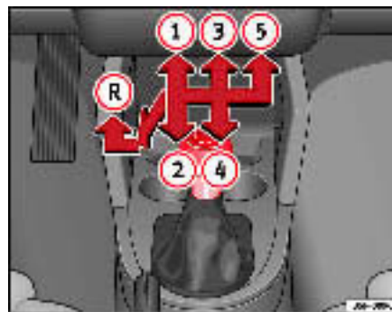
Fig. 136 Détail de la console centrale : schéma d'une boîte de vitesses de 5 marches
