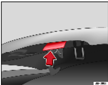
Fig. 161 Gâchette d'ouverture du capot-moteur.
