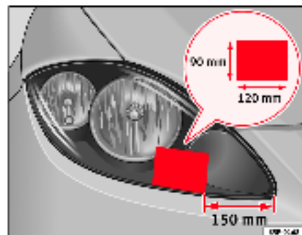
Fig. 150 Phare droit
