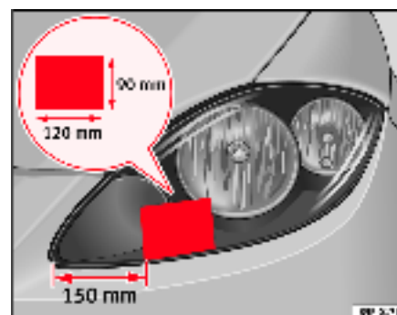
Fig. 153 Phare gauche ▶
