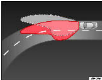
Fig. 76 Éclairage du virage à l'aide des phares autosuggestionner
