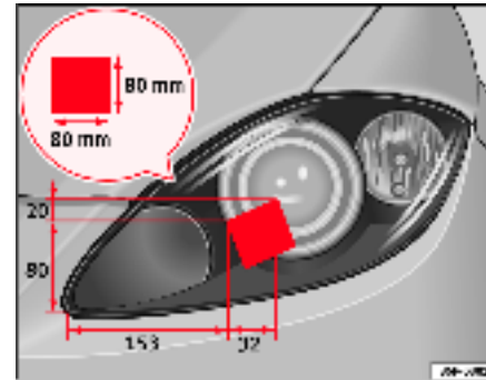
Fig. 155 Phare gauche
