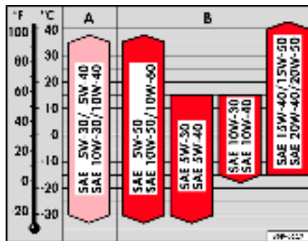
Fig. 162 Types d'huile en fonction de la température
