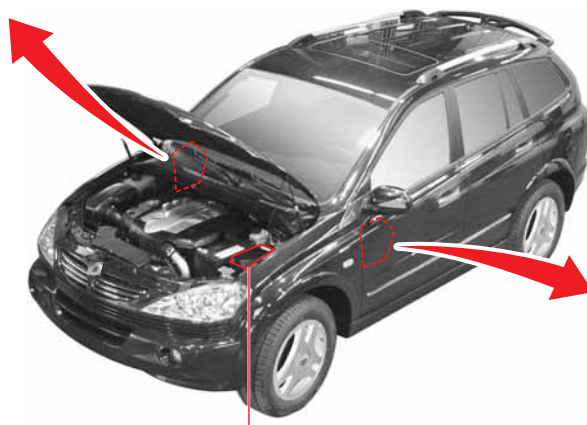
8 Boîte à fusibles et relais du compartiment moteur
