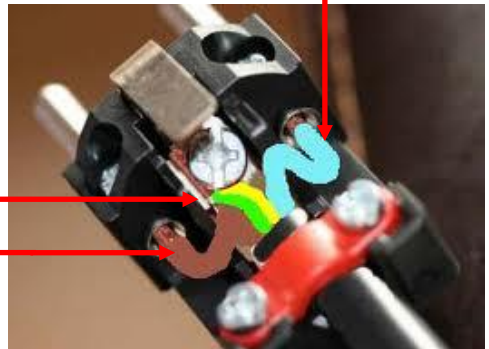
Blauer Draht(N)
