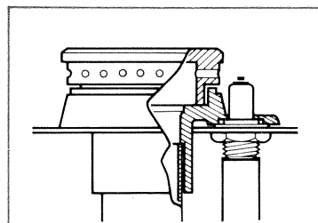
Montage correct de la bougie
